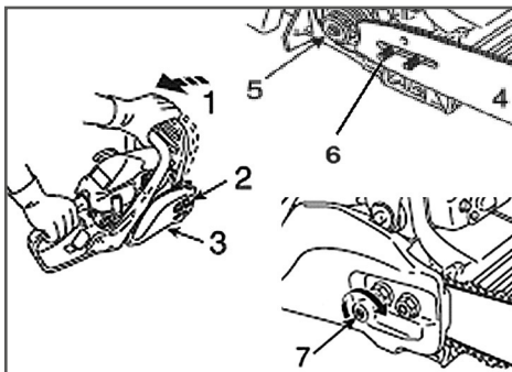
Рис. 2 Установка шины
