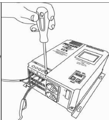
Рис 8. Подключение нагрузки
