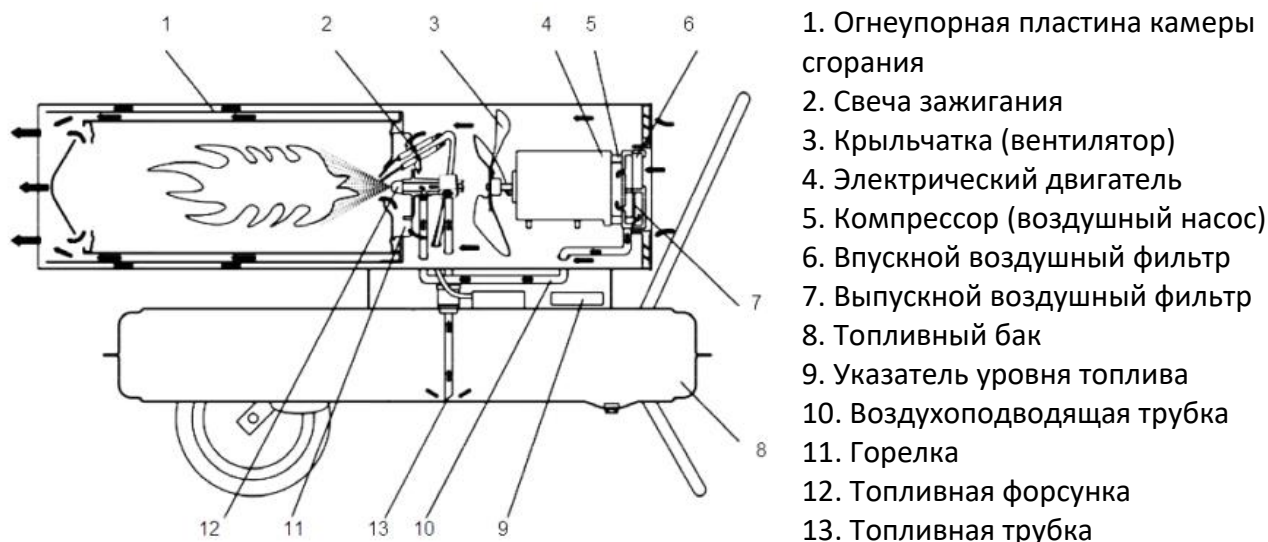
Рис.5 Внутреннее устройство тепловой пушки
