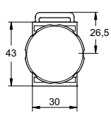
Джойстик
