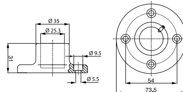
Схема сверления отверстий для сигнальных маяков
