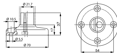
Схема сверления отверстий для сигнальных стоек K70
