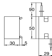
Трансформатор
