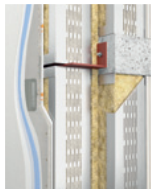
Двухконтурная конструкция стены
